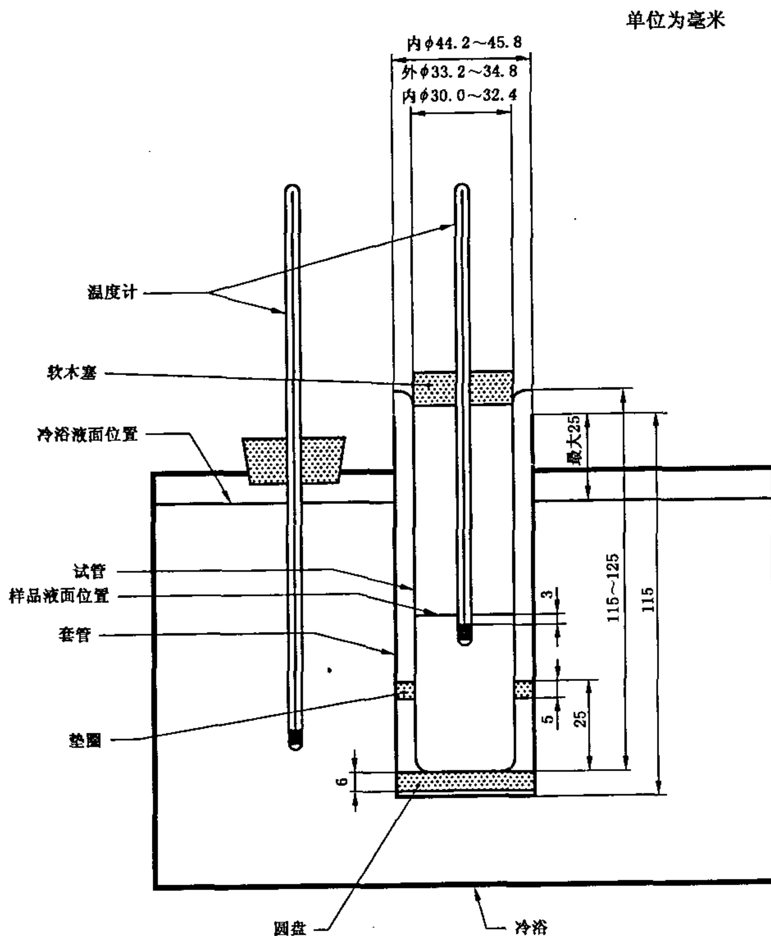
图1 倾点测定仪
